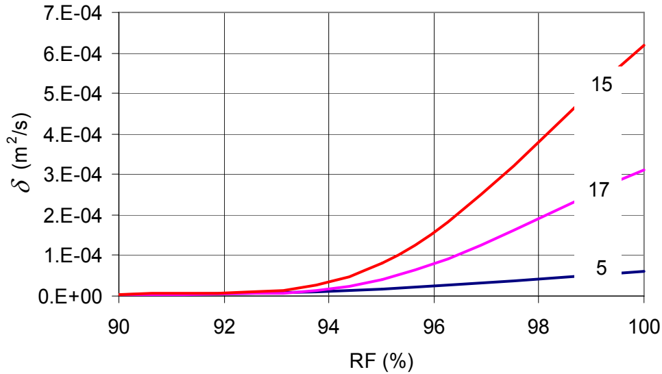
Figur 9.3.6 Fuktransportkoefficienterna för betongen med vct 0.70, med material 5 som utgångspunkt och koefficienterna ökade vid 95 och 100 % RF med faktorerna 2.5 & 5 (material 17) respektive 5 & 10 (material 15). Förstoring i intervallet 90 -100 % RF
